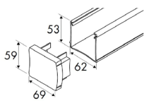
Oberprofil
